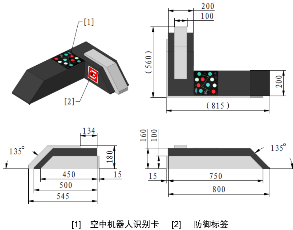
图 2-18 L 地形块示意图
