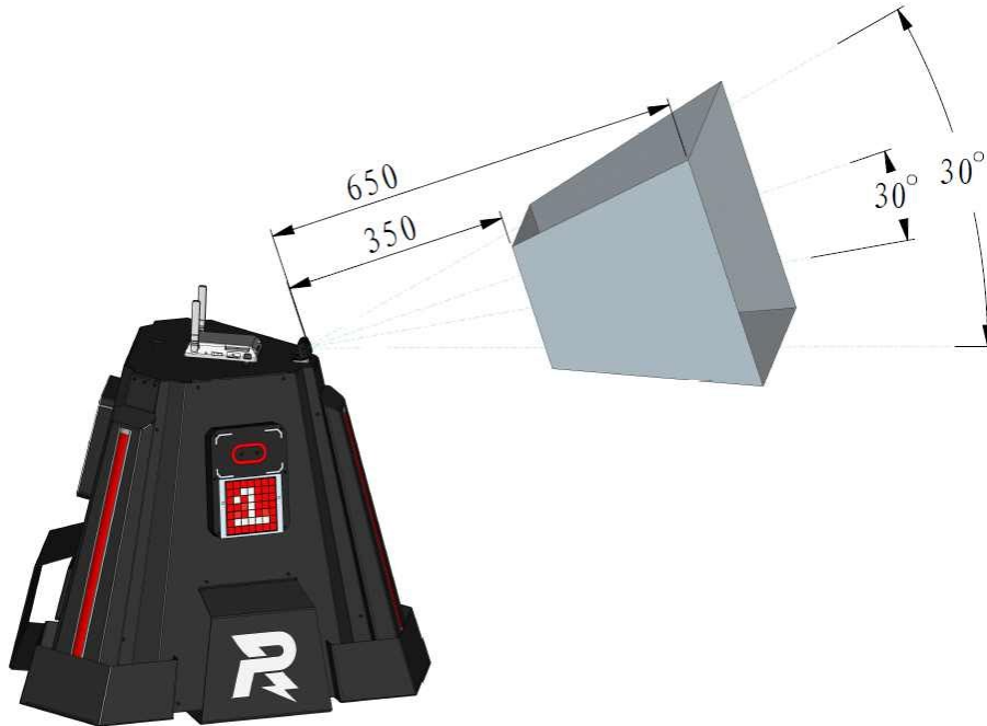
图 3-8 基地识别区示意图
