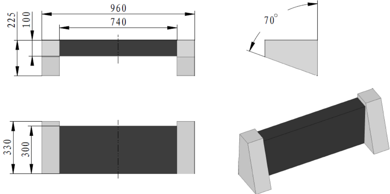
图 2-21 高墙示意图
