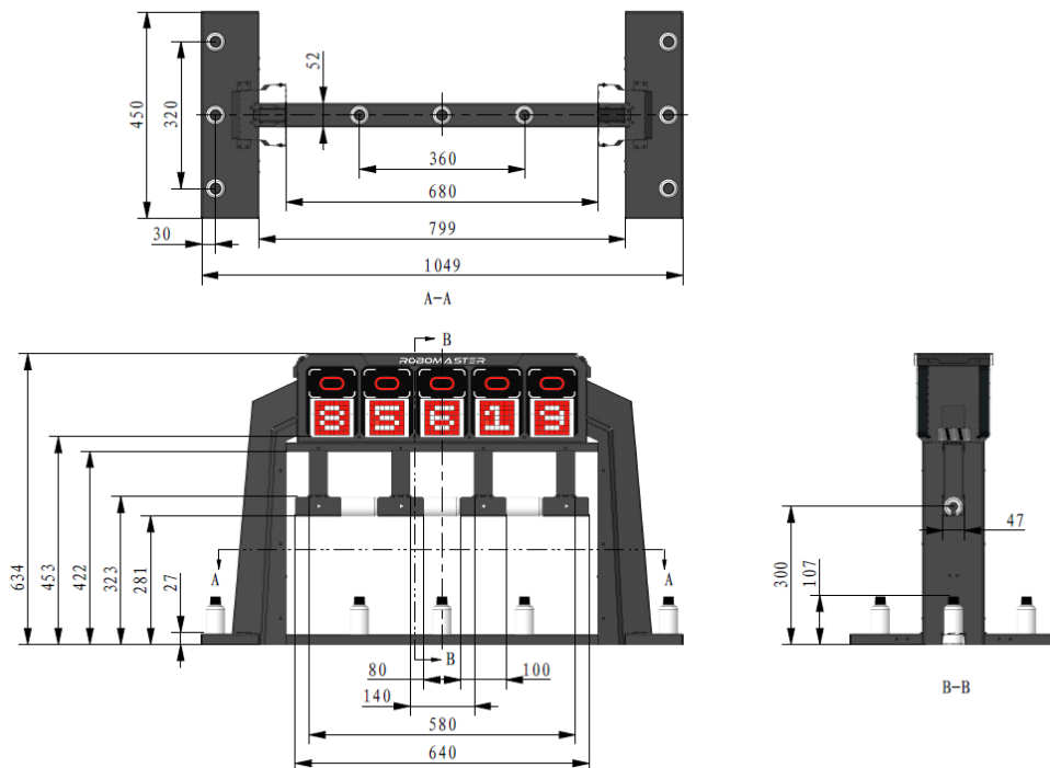
图 2-23 资源岛尺寸图
