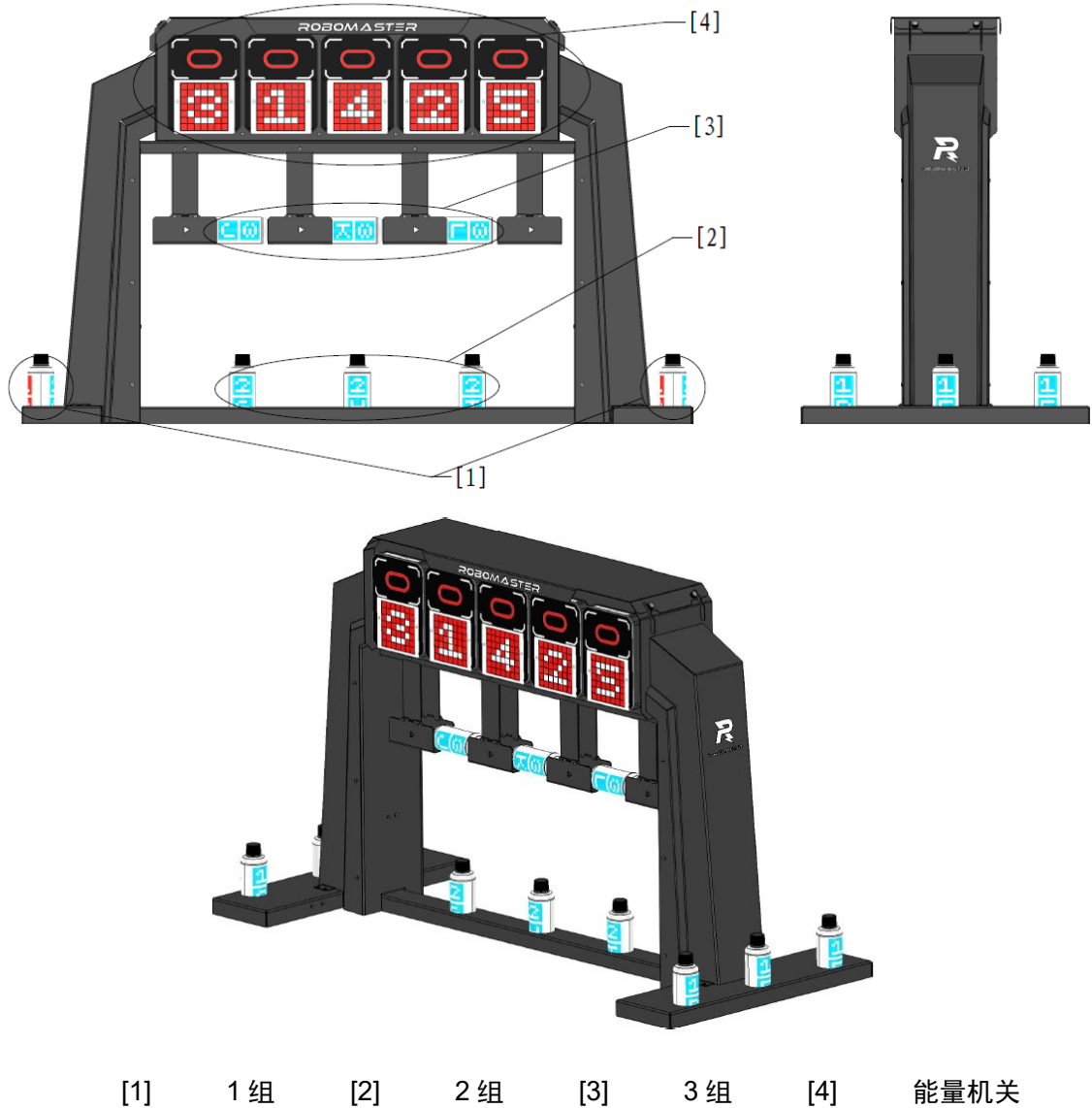
图 3-10 弹药瓶分布示意图
