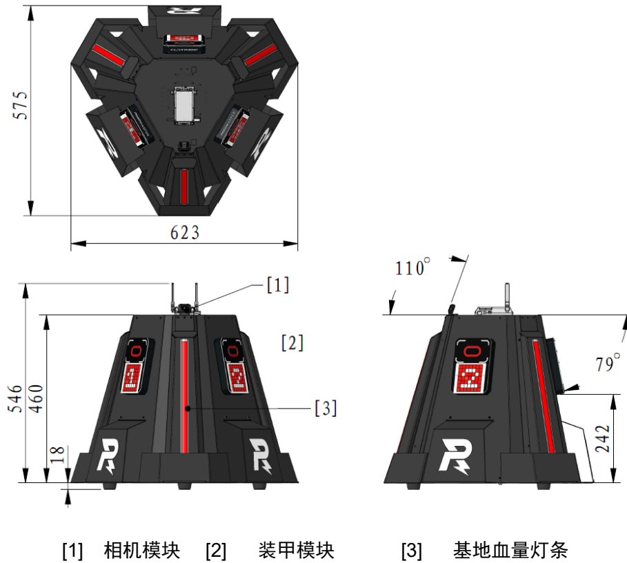
图 2-11 基地示意图
