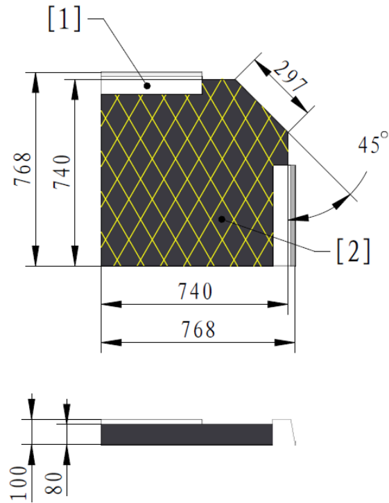
[1] 基地底座 [2] 基地禁区
